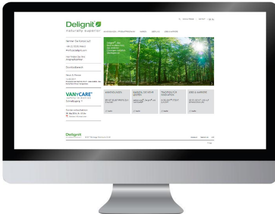
Abbildung 1: Neuer Delignit®-Webauftritt
